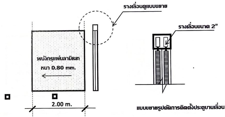
แบบขยาย A06
