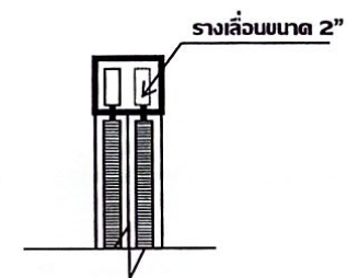
แบบขยายรูปตัดการติดตั้งประตูปานเหล็ก
