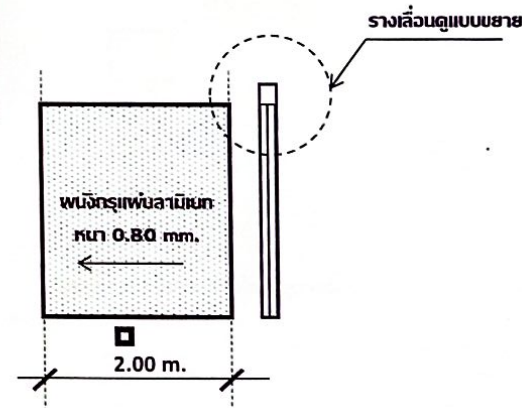
แบบขยายรูปตัดการติดตั้งประตูปานเหล็ก
