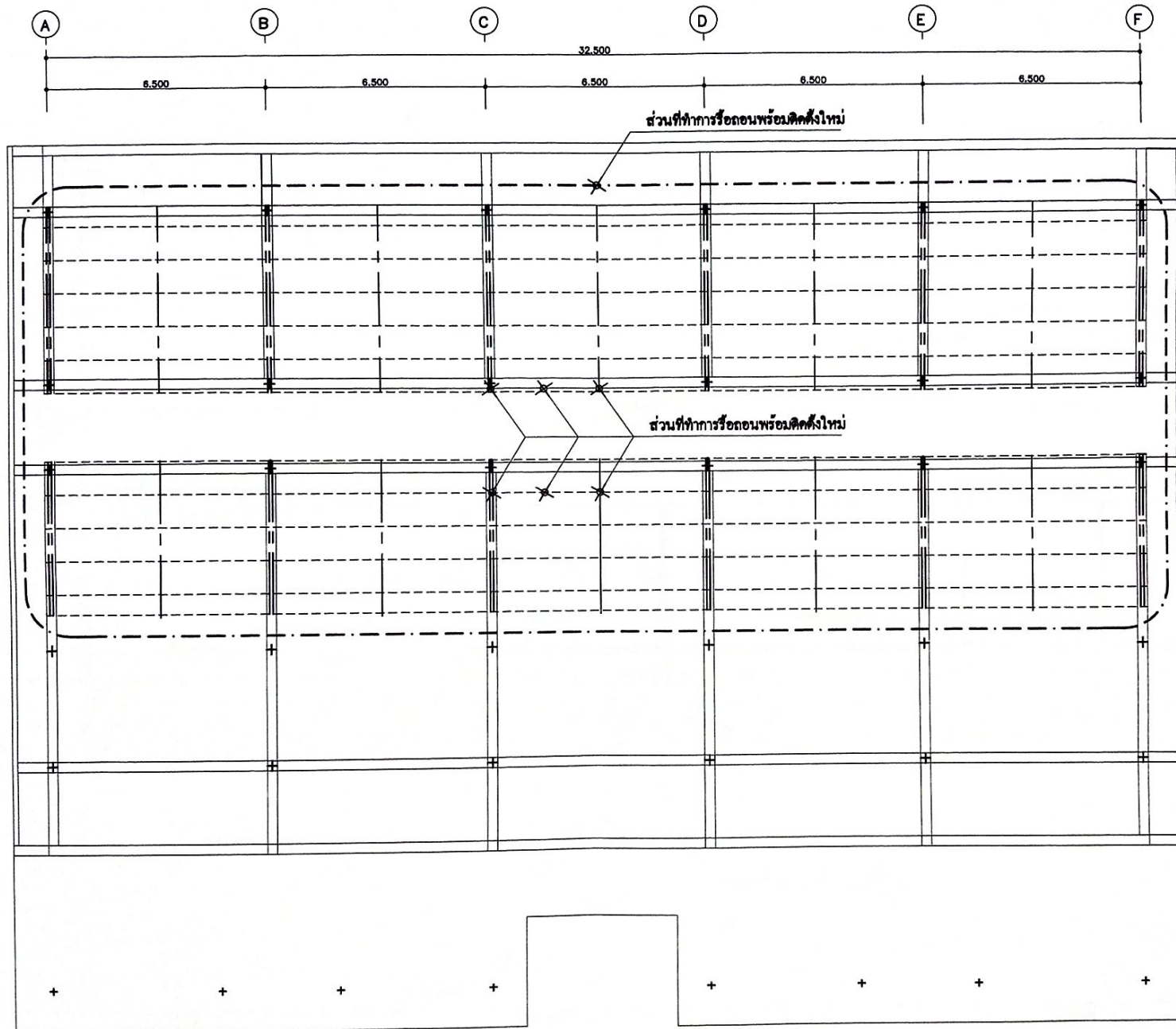
แปลนรื้อถอนโครงสร้างหลังคาเดิม มาตราส่วน 1 : 125
