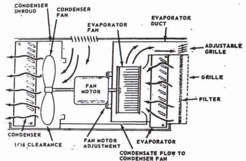
แบบขยายการติดตั้งเครื่องเป่าอากาศ
