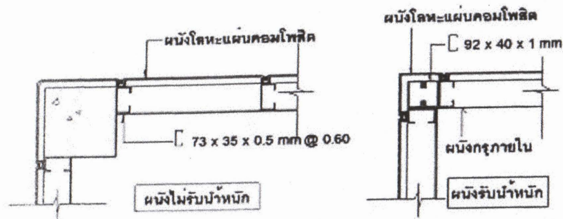
แบบขยายการติดตั้งผนังเบา
